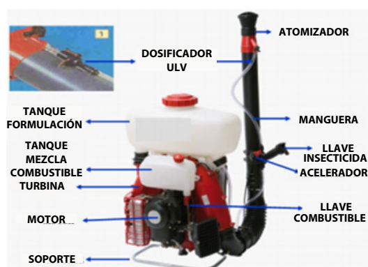
Partes de una máquina motomochila ULV
